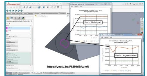
Abb. 1: Verdrillwinkel in Winkelgrad [°] vs. Längeneinheiten [mm]
