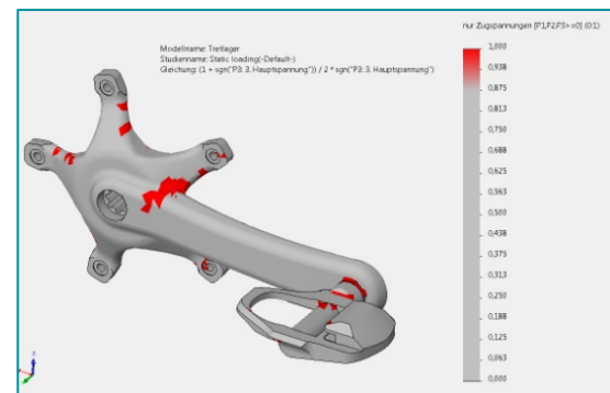
Abb. 3: Geometriebereiche rein auf Zugspannung belastet
