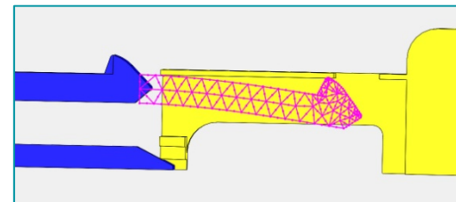
Abb. 2: FEM-Netz in 3D Skizzen umwandeln
