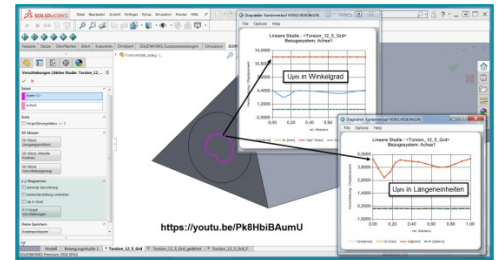
Abb. 1: Torsion in Winkelgrad [°] vs. Längeneinheiten [mm]
